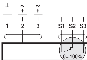
SH24A-S..
