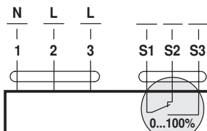
SH230A-S..
