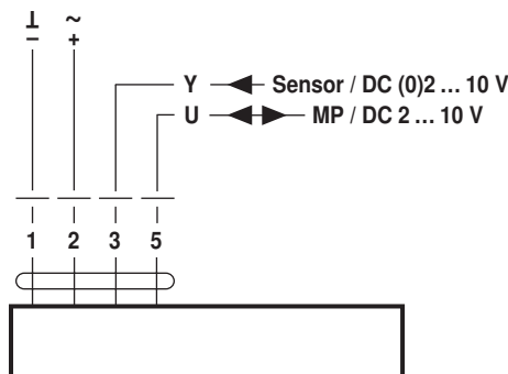
NRF24A-MP(-O) SRF24A-MP(-O)
