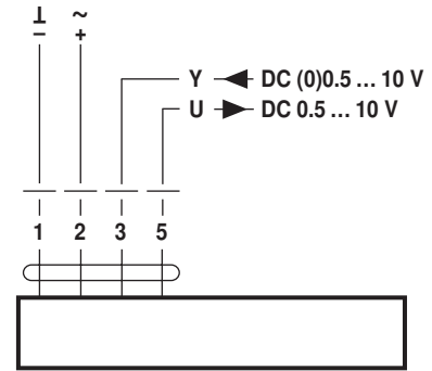
NRF24A-SZ(-O) SRF24A-SZ(-O)
